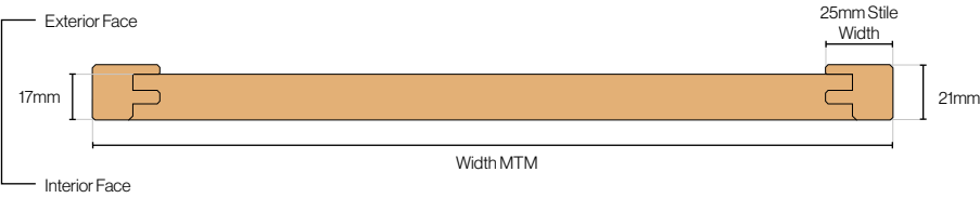
Brooklyn Oak Door Cross Section
