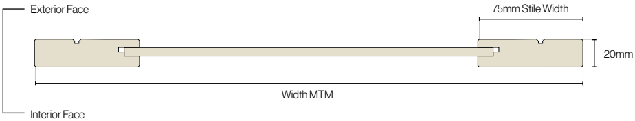
Campbell Door Cross Section
