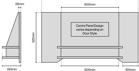
Modern Canopy 1000mm (L) x 193mm (D) x 525mm (H)
