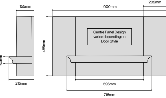
Classic Canopy 1000mm (W) x 215mm (D) x 485mm (H)
