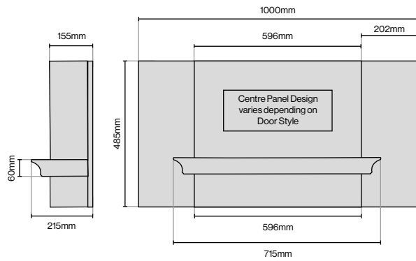
Classic Canopy 1000mm (W) x 215mm (D) x 485mm (H)
