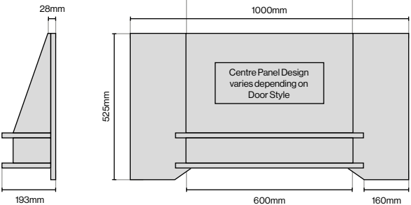
Modern Canopy 1000mm (W) x 193mm (D) x 525mm (H)
