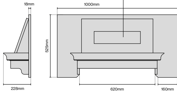
Modern Canopy 1000mm (W) x 228mm (D) x 525mm (H)
