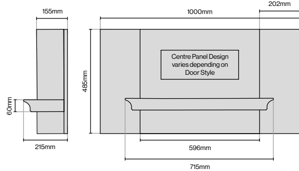
Classic Canopy 1000mm (W) x 215mm (D) x 485mm (H)
