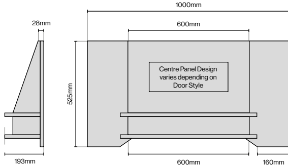
Modern Canopy 1000mm (L) x 193mm (D) x 525mm (H)
