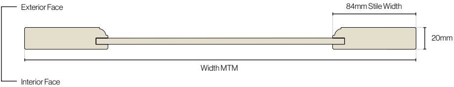
Edison Door Cross Section
