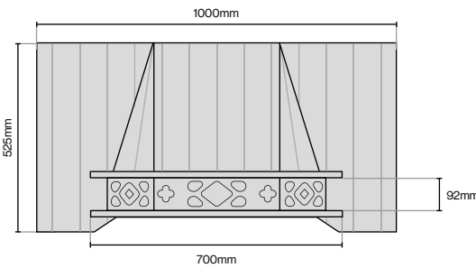
Traditional Canopy* 1000mm (L) x 193mm (D) x 525mm (H)
