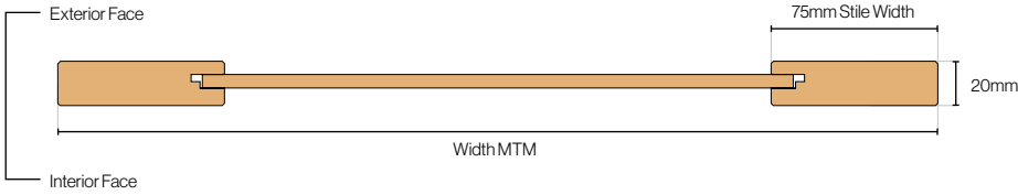
Monroe Oak Door Cross Section
