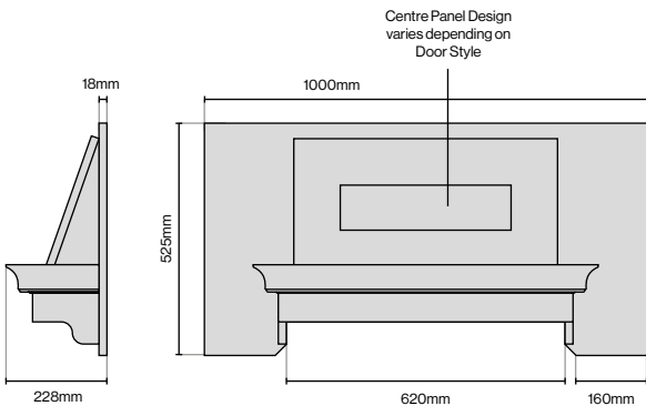
Modern Canopy 1000mm (W) x 228mm (D) x 525mm (H)
