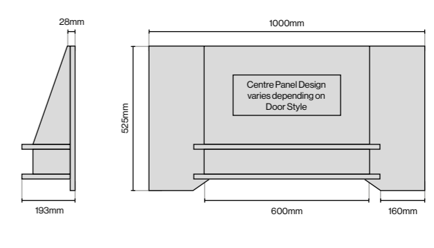
Modern Canopy 1000mm (W) x 193mm (D) x 525mm (H)
