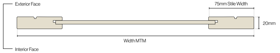
Campbell Door Cross Section
