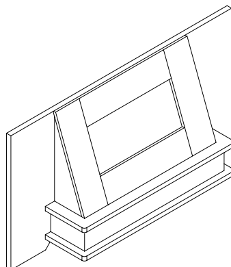
Modern Canopy 1000mm (L) x 193mm (D) x 525mm (H)
