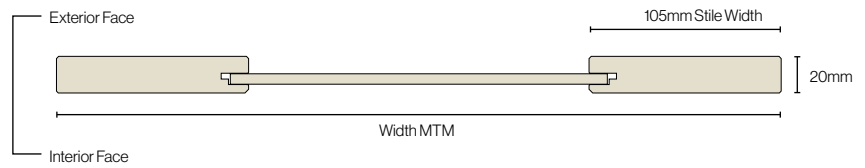
Albany Door Cross Section
