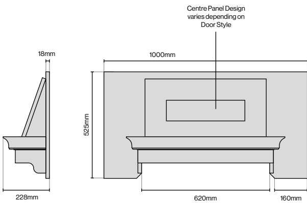
Modern Canopy 1000mm (W) x 228mm (D) x 525mm (H)
