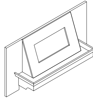
Modern Canopy 1000mm (W) x 228mm (D) x 525mm (H)
