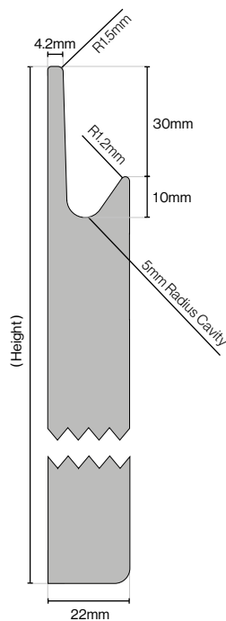
Arena Door Cross Section
