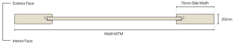
Monroe Door Cross Section
