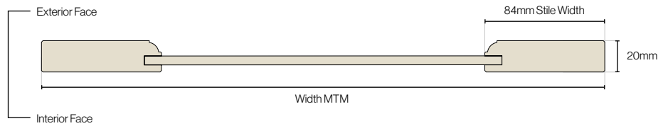
Edison Door Cross Section
