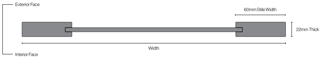
Harlem Door Cross Section
