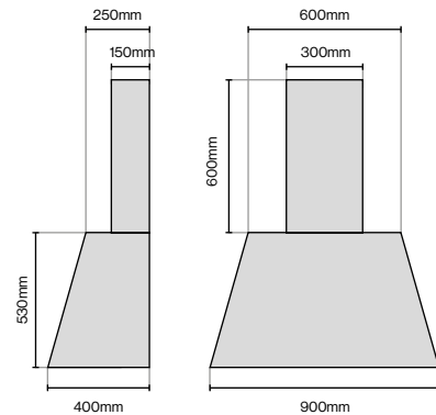
Chimney Canopy 900mm (W) x 400mm (D) x 1130mm (H)
