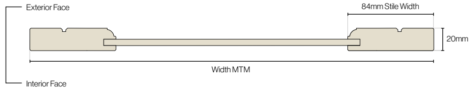
Rainey Door Cross Section
