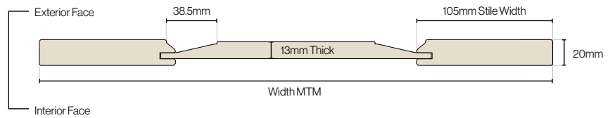
Hampton Door Cross Section
