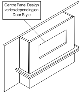
Classic Canopy 1000mm (W) x 193mm (D) x 525mm (H)
