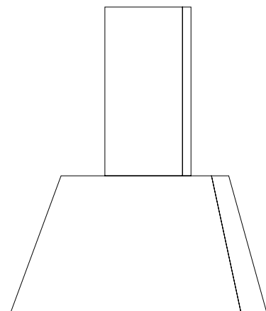
Chimney Canopy 900mm (W) x 400mm (D) x 1130mm (H)
